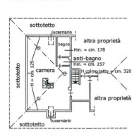
Piano Secondo (Sottotetto) Hm. = cm. 222
